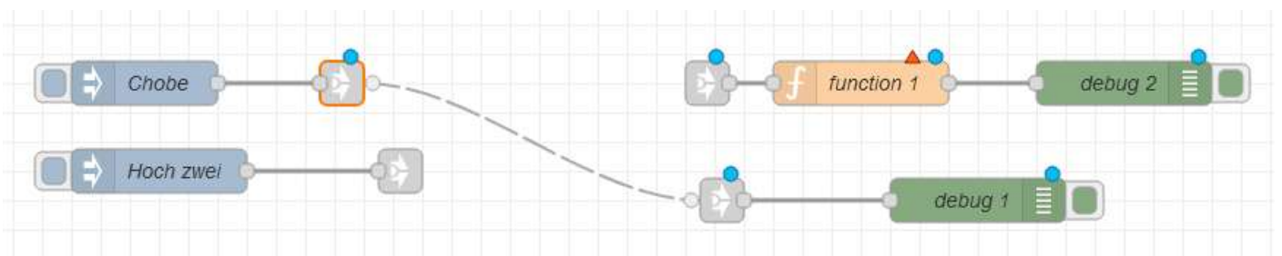
sichtbare Verbindung zweier Nodes mit link-in/link-out
