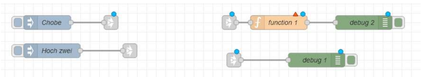
unsichtbare Verbindung zweier Nodes mit link-in/link-out
